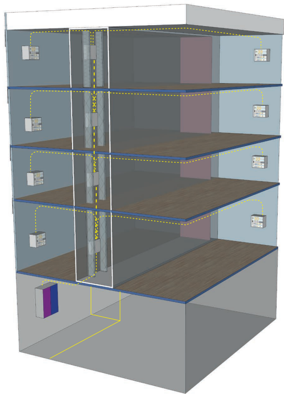
Fig 51 : Exemple de distribution FttH d'un immeuble de bureaux
